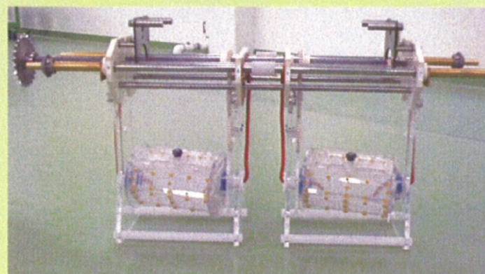
自動機仕様2連型バレル (BFバタフライ型アミ張りタイプ)
